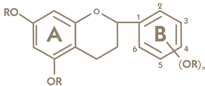
Actividad Antioxidante del Bambú. Estructura general de los flavonoides
